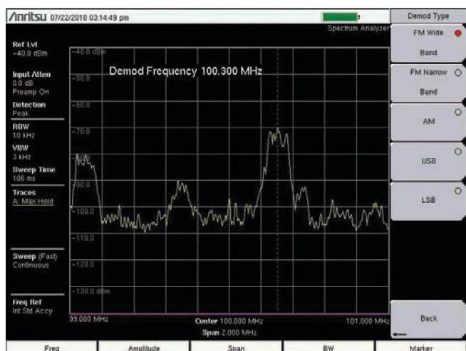
Демодуляция AM/ЧМ/ОБП
