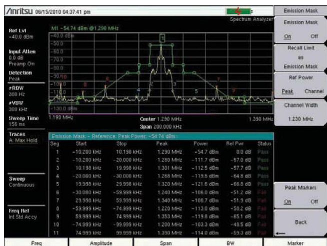
Маска излучения
