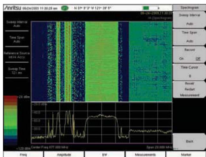
Спектрограмма
