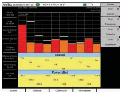
Сканер каналов
