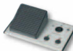
CM 4120 F Пульт Председателя, настольный, встроенный громкоговоритель, с разъемом XLR для микрофона
