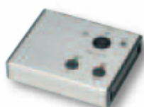
CM 4121 P Пульт Председателя, настольный, с разъемом XLR для микрофона
